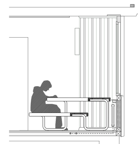
Schnitt 1:50
