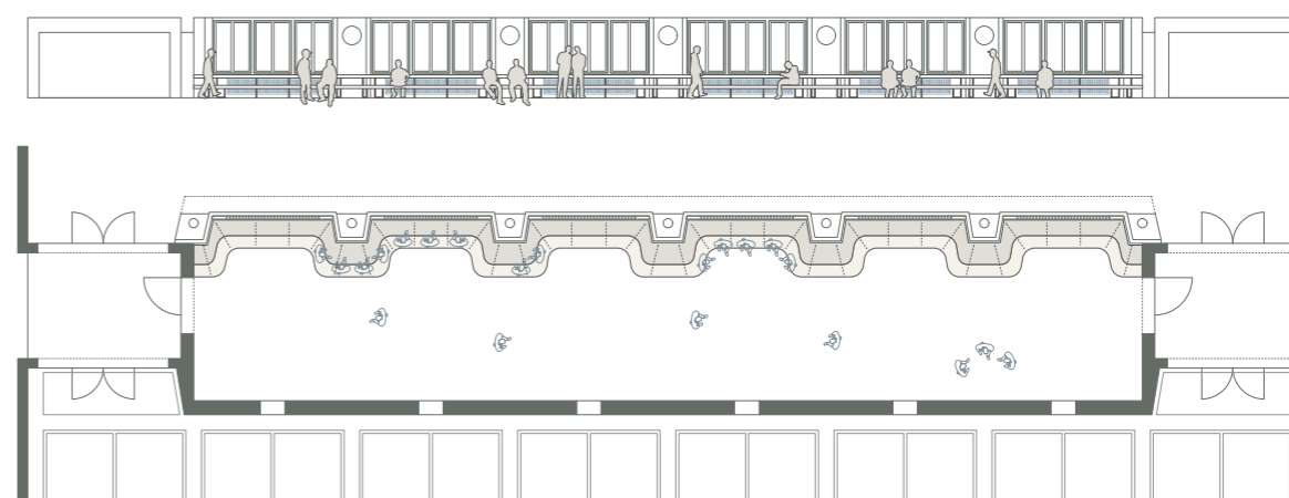
Ansicht und Grundriss Milchhalle 1:150
